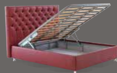
Capacità versioni UP con Piano Letto Classic B3 . Ring Medium Altezza Interna: 12 cm. Volume 400 litri. Ring Large Altezza Interna: 18 cm. Volume 550 litri. Ring Extra Large Altezza Interna: 24 cm. Volume 750 litri.
