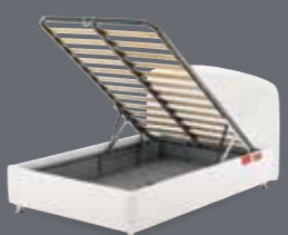
Capacità versioni UP con Piano Letto Classic D3 . Ring Medium Altezza Interna: 12 cm. Volume 300 l. Ring Large Altezza Interna: 18 cm. Volume 420 l. Ring Extra Large Altezza Interna: 24 cm. Volume 550 l.
