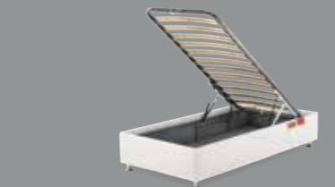
Capacità versioni UP con Piano Letto Classic G3 . Ring Medium Altezza Interna: 12 cm. Volume 200 l. Ring Large Altezza Interna: 18 cm. Volume 275 l. Ring Extra Large Altezza Interna: 24 cm. Volume 375 l.
